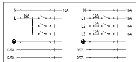
Schema elettrico Electrical scheme
